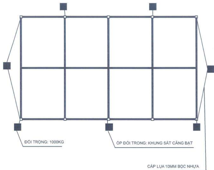
VỊ TRÍ ĐẶT ĐỐI TRỌNG
