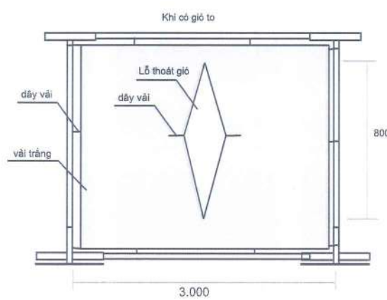
PHƯƠNG ÁN THI CÔNG HÀNG RÀO
