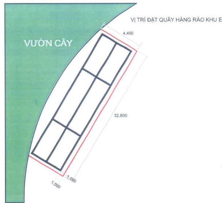
PHƯƠNG ÁN THI CÔNG HÀNG RÀO
